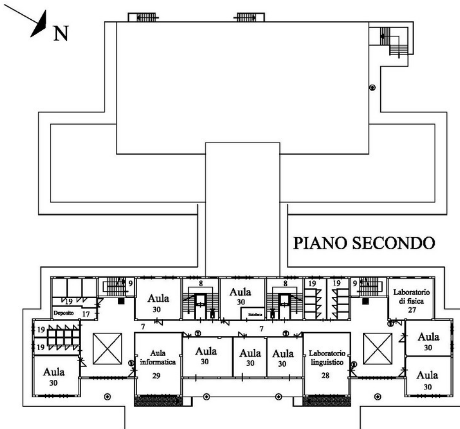
Planimetria piano SECONDO
